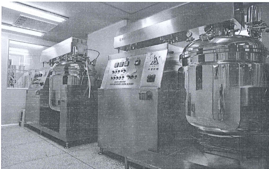
凝胶配料锅
