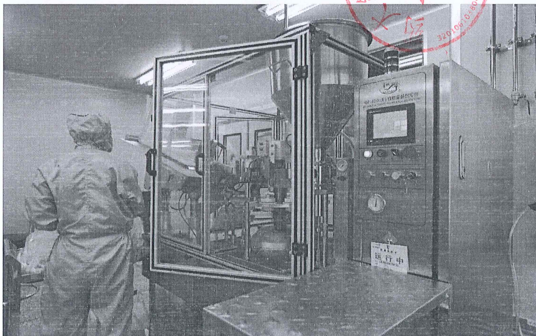
凝胶自动灌装封尾机
